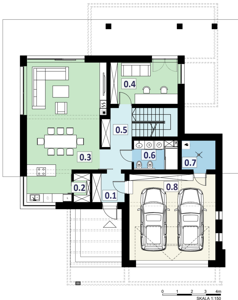
RZUT PARTERU
