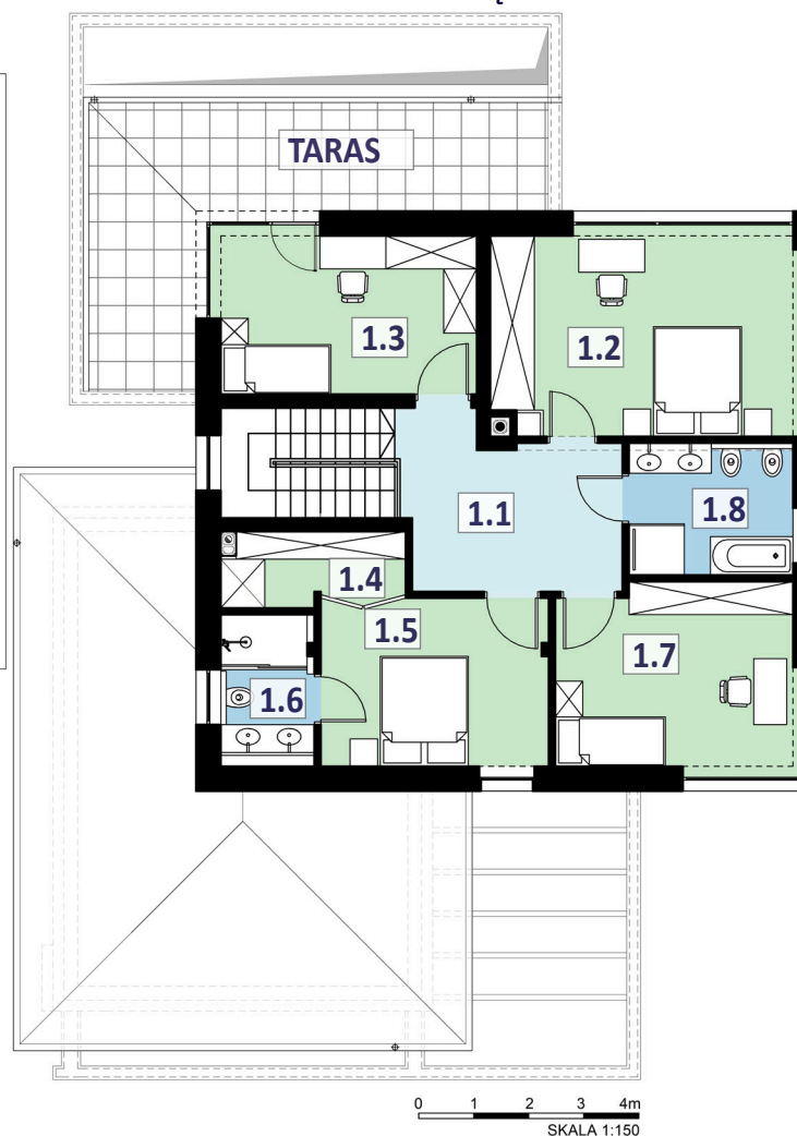
RZUT 1 PIĘTRA
