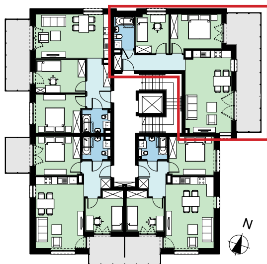
RZUT 1 PIĘTRA LOKALIZACJA MIESZKANIA
