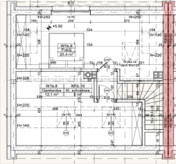
Rzut mieszkania · Drugie piętro
