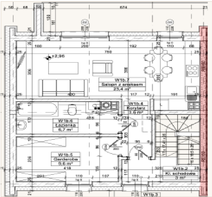
Rzut mieszkania · Parter i pierwsze piętro
