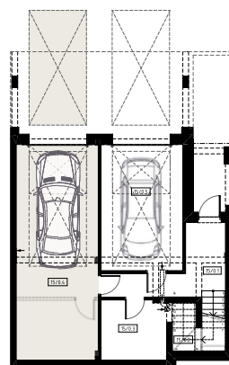
rzut poziomu 0
