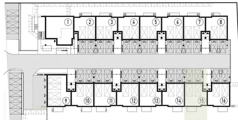
rzut poziomu 2
