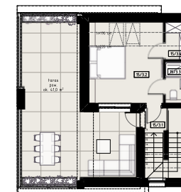
rzut poziomu 3
