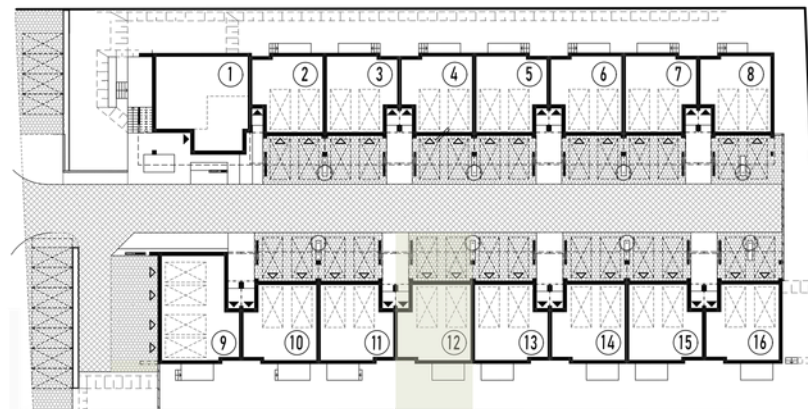
rzut poziomu 2
